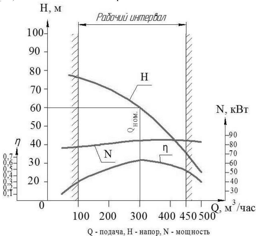
Рисунок 1 - Характеристики насоса ОДН 300-200-150, насосной установки УОДН 300-200-150-90 на воде.
