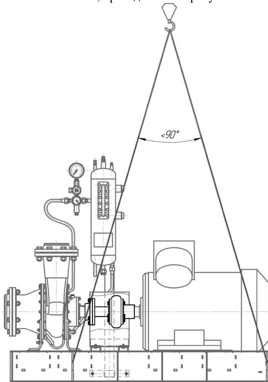
Рисунок 5- Схема строповки
