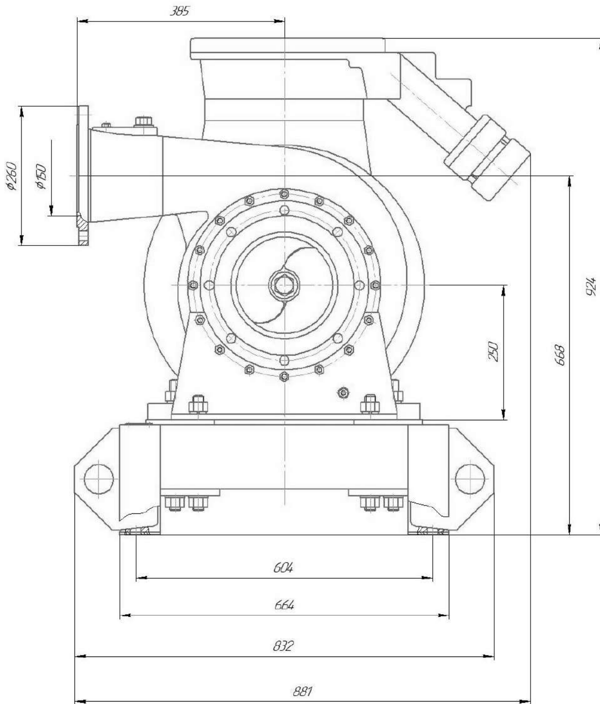
Рисунок 2а - Устройство насосной установки УОДН 300-200-150-90-ТД
