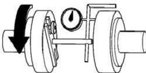
Рисунок 7 - Проверка углового смещения
